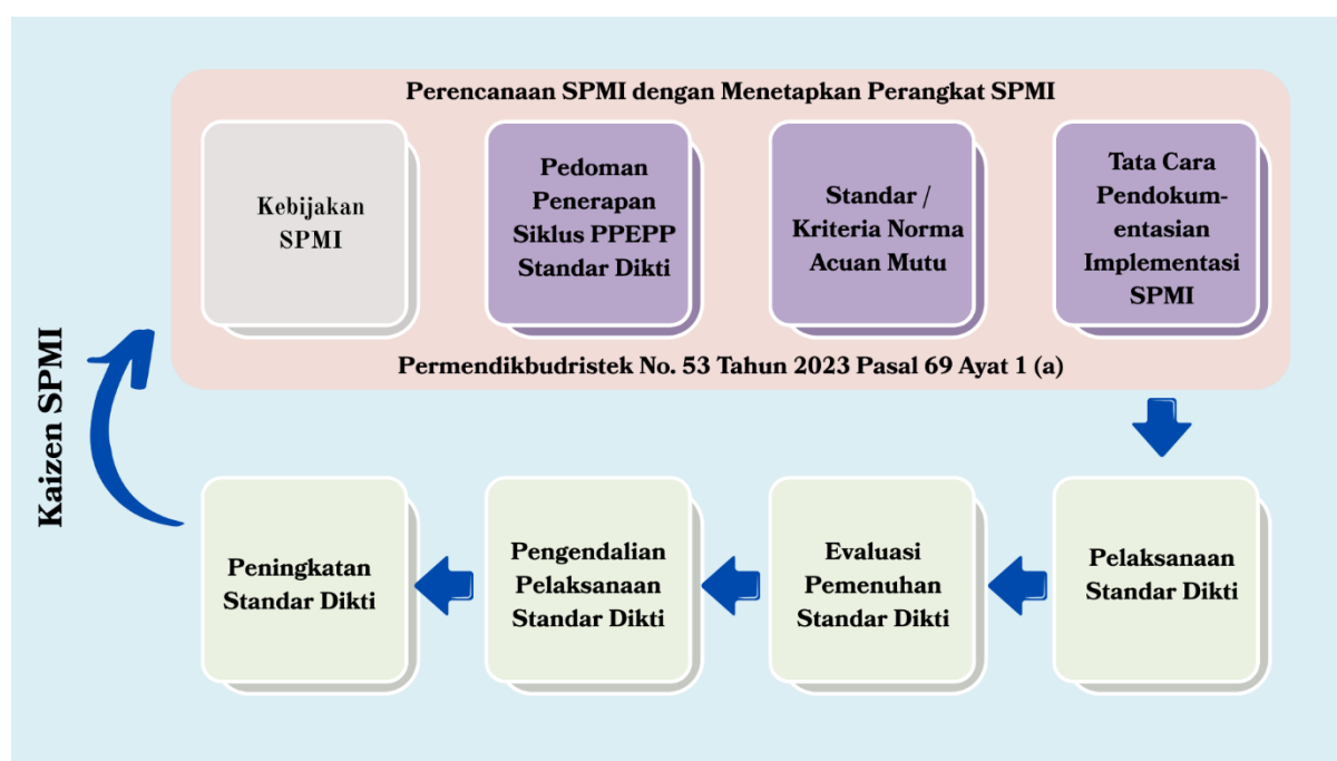
Gambar 9. Implementasi SPMI
